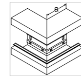
Külső sarok Alumínium
