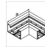
Függőleges sarokelem Alumínium
