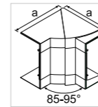
Állítható belső sarok PC - ABS
